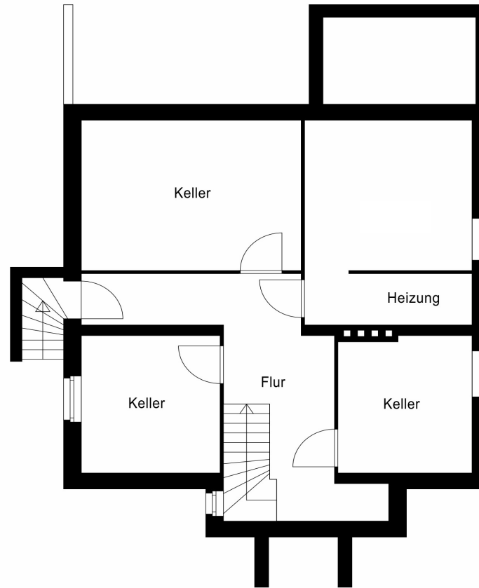
Kellergeschoss
